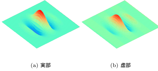
図 1 2次元 Gabor フィルタの概観。 Fig. 1 An overview of 2D Gabor filters.
