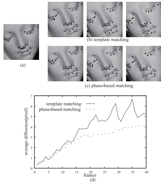
図 8 物体が姿勢変化した画像間の対応付けの結果。(a) が基準画像、(b) がテンプレートマッチング (正規化相関) による対応付け、(c) が位相を利用した手法による対応付けの結果の例である。(d) は基準画像上でのエビポーラ線と対応点の距離の平均を表す。
