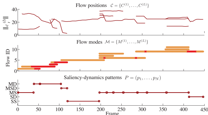
図3 顕著性変動の解析。上段: 各 Saliency flow の重心位置の変化 (縦軸は画像左上を原点にとった重心位置のノルム)、中段: 各 Saliency flow のモード (赤: 動的状態, 橙: 静的状態)、下段: 顕著性変動パターン (SS: Single Static, SD: Single Dynamic, MS: Multi Static, MSD: Multi Static/Dynamic, MD: Multi Dynamic)。各パラメータは \pi_c = 2^\circ/\text{s} , \omega_d = 2^\circ , w_s = 0.1 \text{ sec} , \omega_p = 0.5 \text{ sec} に設定した。
