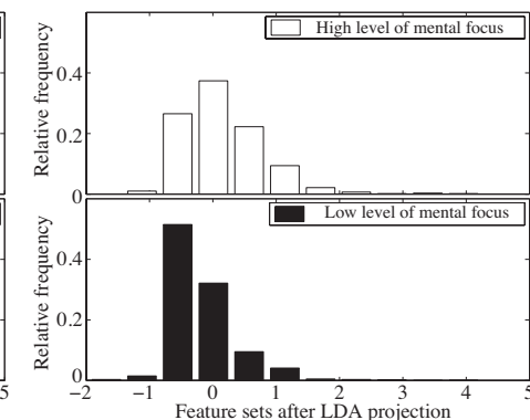
図 8 獲得された相対頻度分布 (MSD)。
